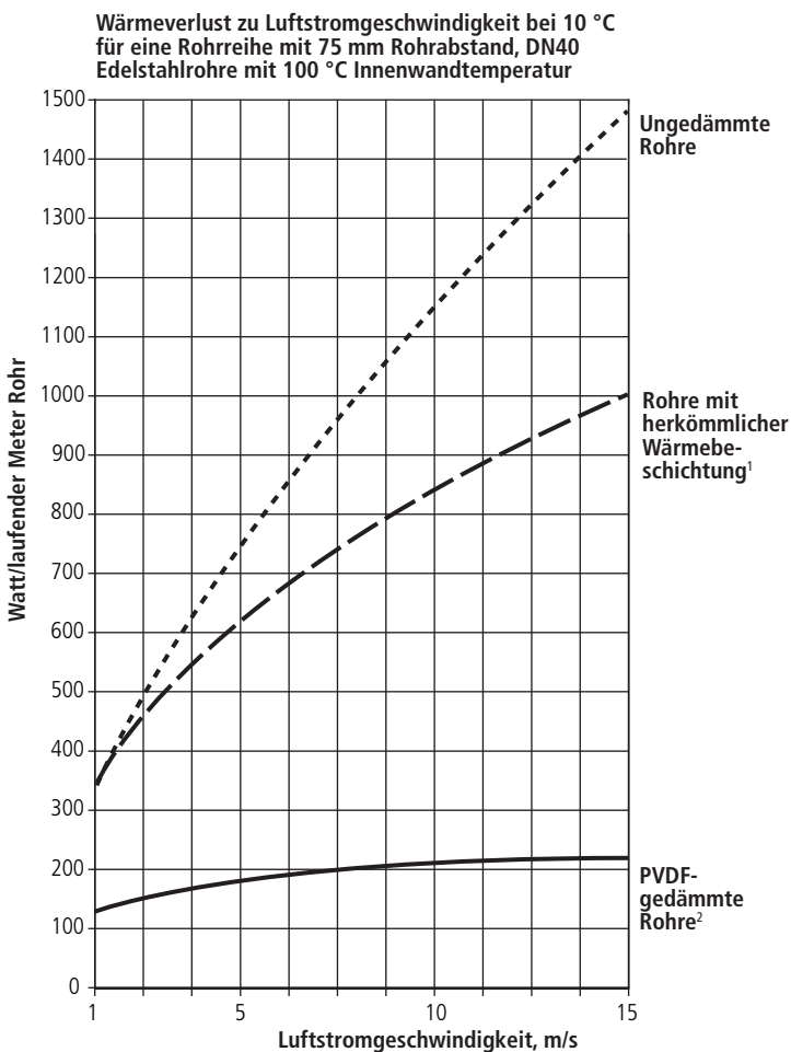
Abbildung 5-1: Verteilrohr-Wärmeabgabe
