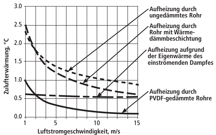
Abbildung 12-1: Aufheizung der Zuluft durch Dampf und durch das Verteilmodul, wie beschrieben in der Musterberechnung auf Seite 7
