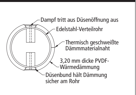
Abbildung 3-1: Querschnitt eines PVDF-gedämmten Verteilrohrs
