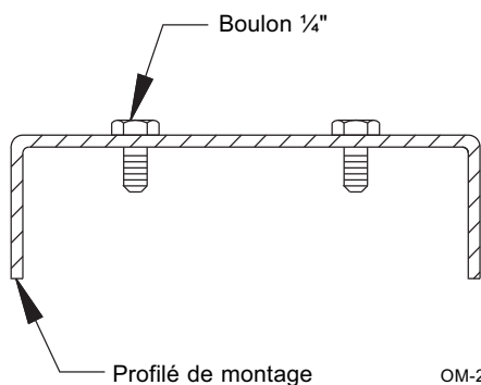
Figure 4-2 : Vue détaillée du profilé de montage
